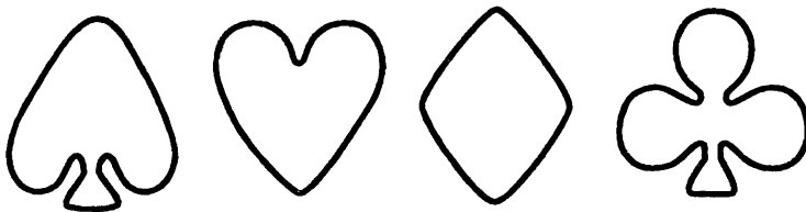
図 14: 単純閉曲線
